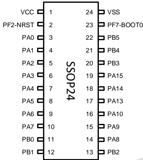
图 3-1 SSOP24 Pinout1 PY32M031E1xT
